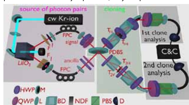
Schéma univerzálního klonovacího zařízení kvantových stavů fotonů. Experiment se skládá ze tří částí – zdroj fotonových párů, klonovací část a dvoufotonová polarizační analýza.
